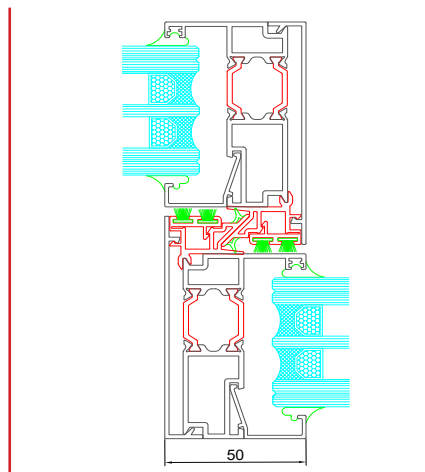
Sección nudo central
