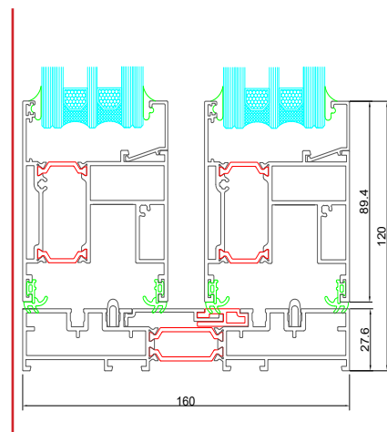
Sección vertical
